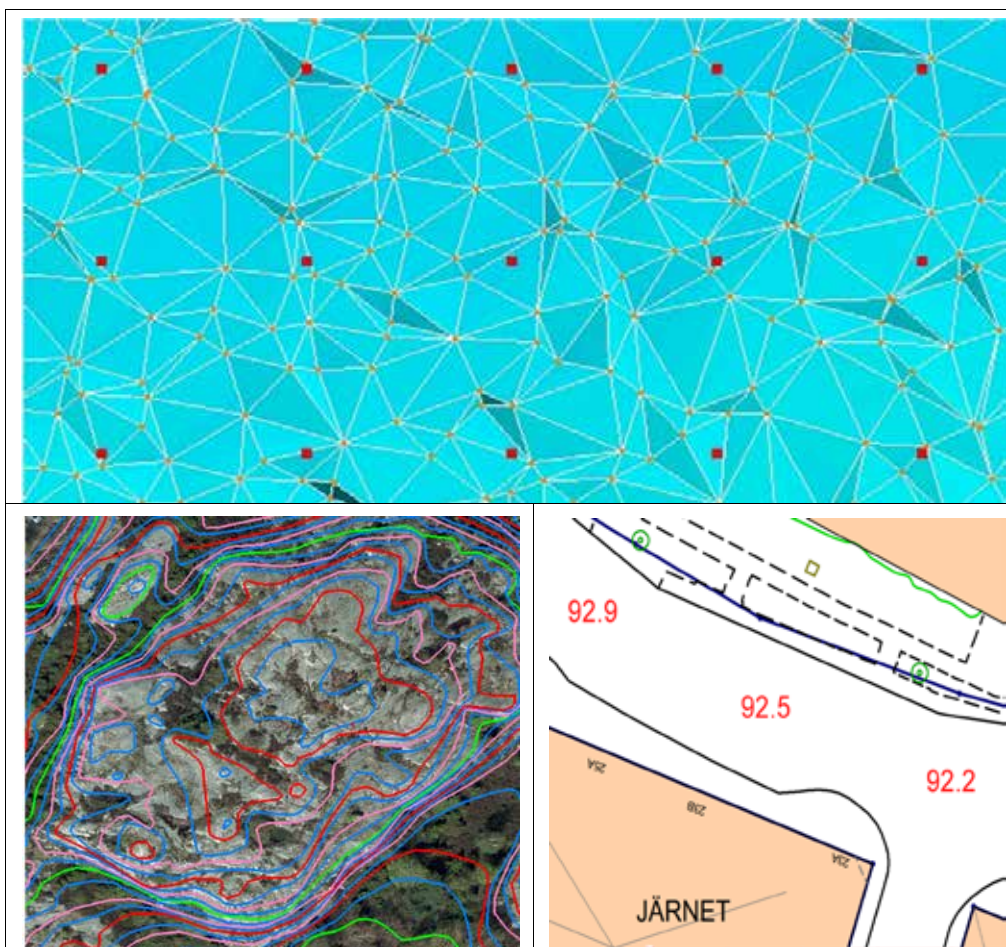
Figur C.2.1a. Exempel på markmodell i form av grid (regelbundna punkter i rött) och TIN (triangelnät baserat på gula punkter), nivåkurvor med 0.5 m ekvidistans och punkthöjder på vägar (röda siffror).
