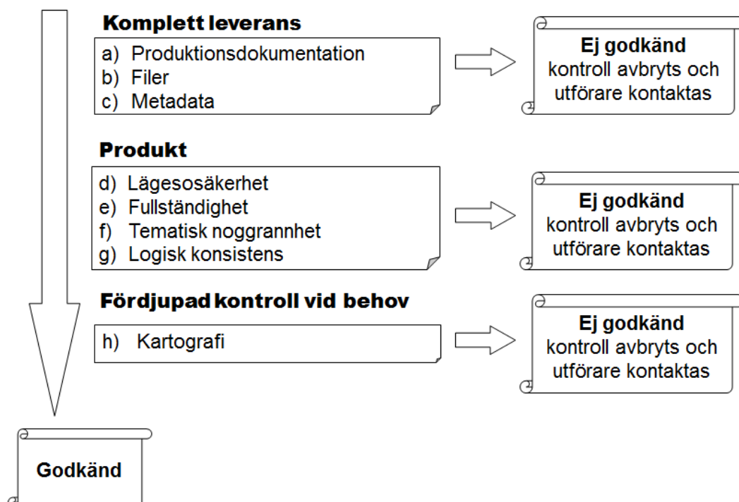
Figur 4. Visualisering av kontrollflödet och de ingående kontrollerna.
