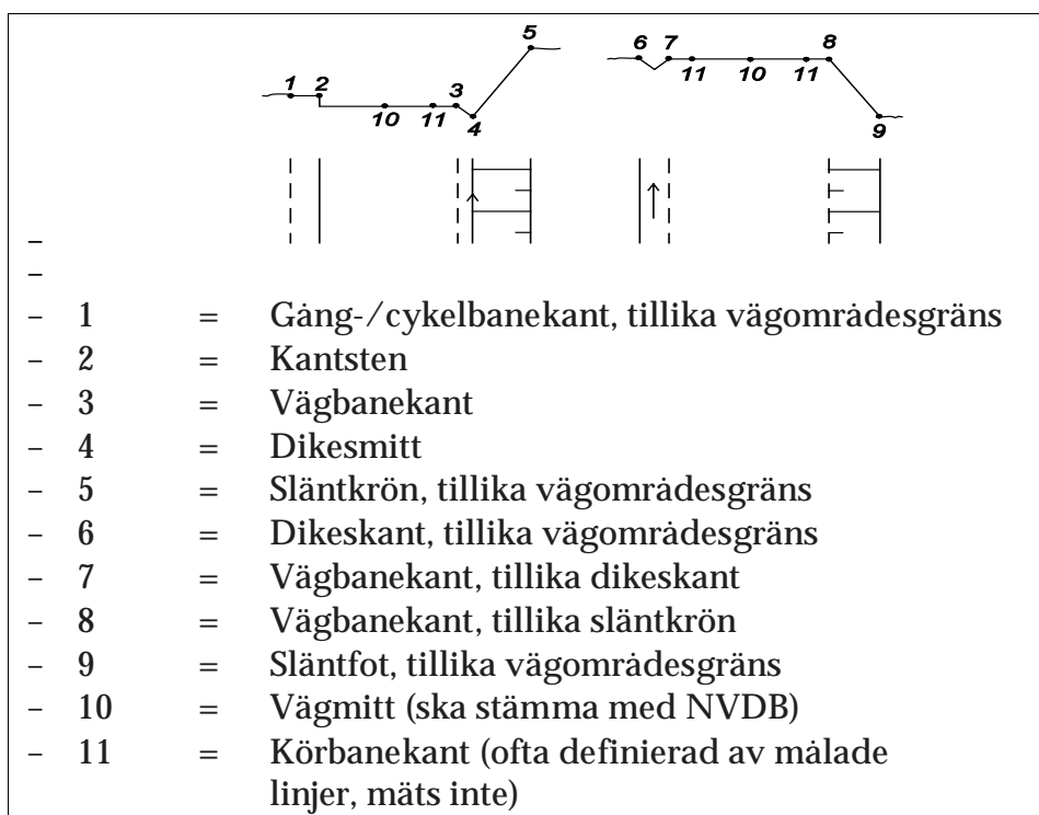
Figur C.2.4a. Anvisning för mätning av vägbana i anslutning till dike, slänt/skärning och gång-/cykelbana. Bildens övre del visar en tvärsektion och den undre delen visar motsvarande område i plan.
